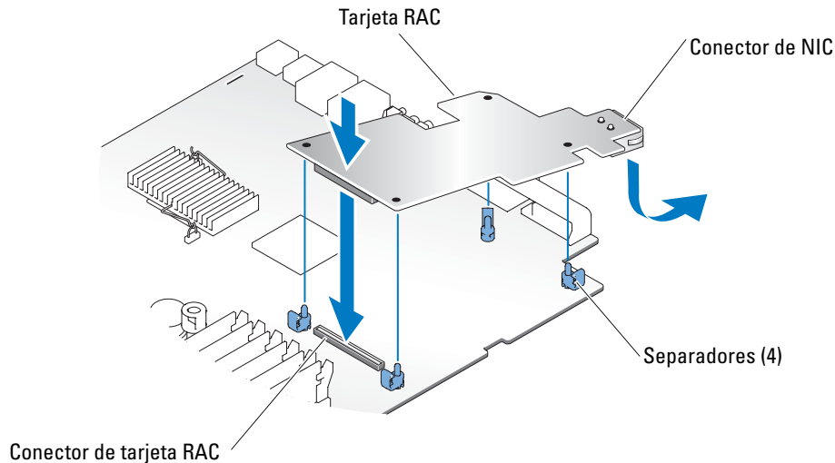
Figura 2. Instalación de una tarjeta RAC
