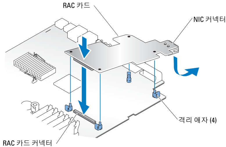
그림 2. RAC 카드 설치
