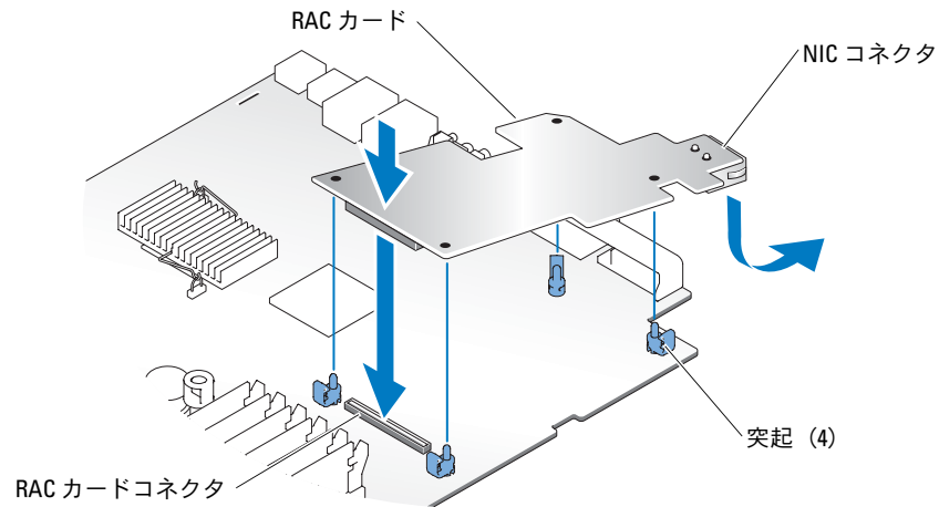
図 2. RAC カードの取り付け
