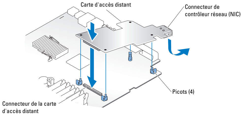
Figure 2. Installation d'une carte d'accès distant
