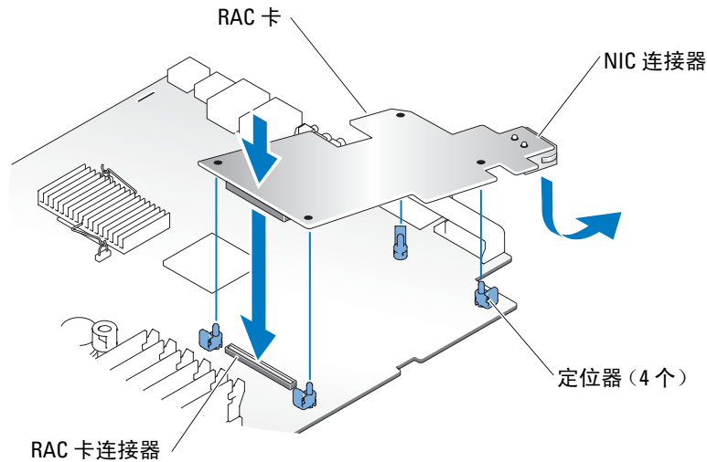
图 2. 安装 RAC 卡
