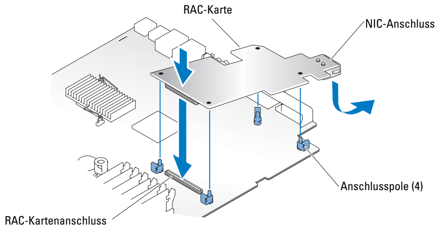
Abbildung 2. RAC-Karte installieren
